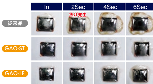
450°Cでの焦げ付き度合比較
