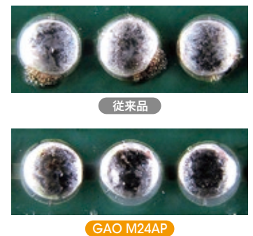
気泡の残存量比較
