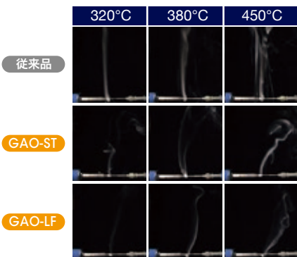
各温度での発煙量比較
